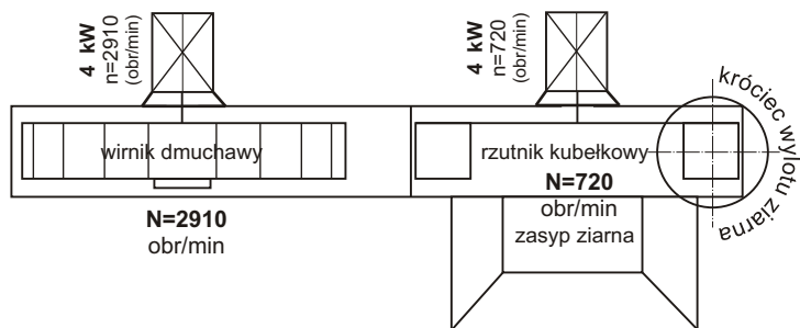
Rys. 4 Schemat napędu przenośnika.
